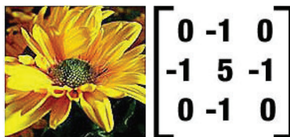
Jc`bX+#) I Primjena filtra za izoštrjenje slike (engl. sharpen ). (preuzeto s poveznice http://designstacks.net/convolution-matrix )
