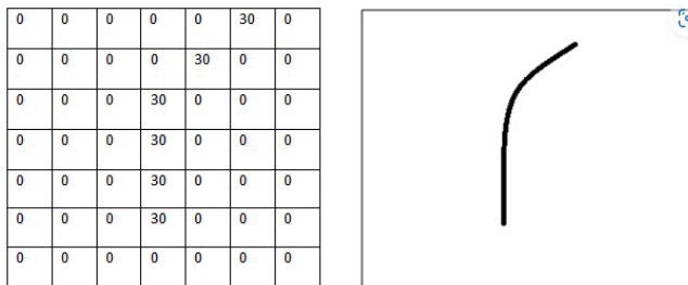
Jc bX+#. I Konvolucijski filtar, u numeričkom i grafičkom zapisu (preuzeto s bloga Adita Deshpandea)
