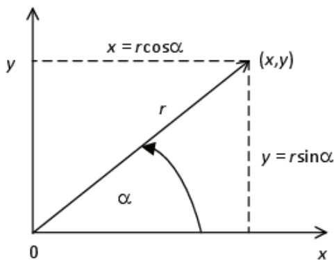
Jc`bX+#(I Vektor (x,y) u polarnom koordinatnom sustavu.
