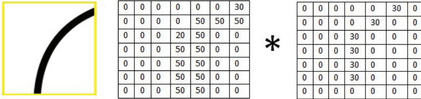
Jc'bx+#0I Receptivno polje s prethodne slike, njegova numerička reprezentacija i numerička reprezentacija filtera. (preuzeto s bloga Adita Deshpanda)
