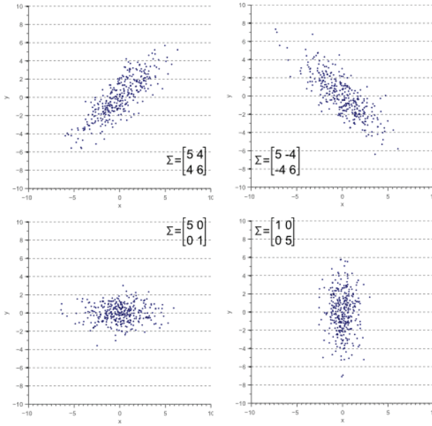
Jc`bX+70I Skup podataka iz vizure kovarijanci (gornji red) i varijanci (donji red) (preuzeto s poveznice https://www.visiondummy.com/2014/04/geometric-interpretation-covariance-matrix/ )
