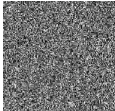
Jc`bX+#' I Bijeli šum
