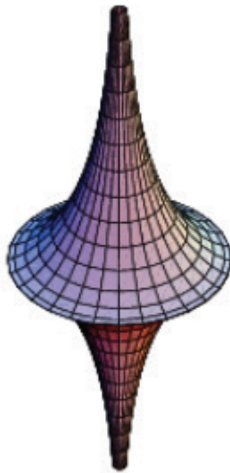
Jc`bX+#( IPseudosfera-model hiperboličke geometrije
