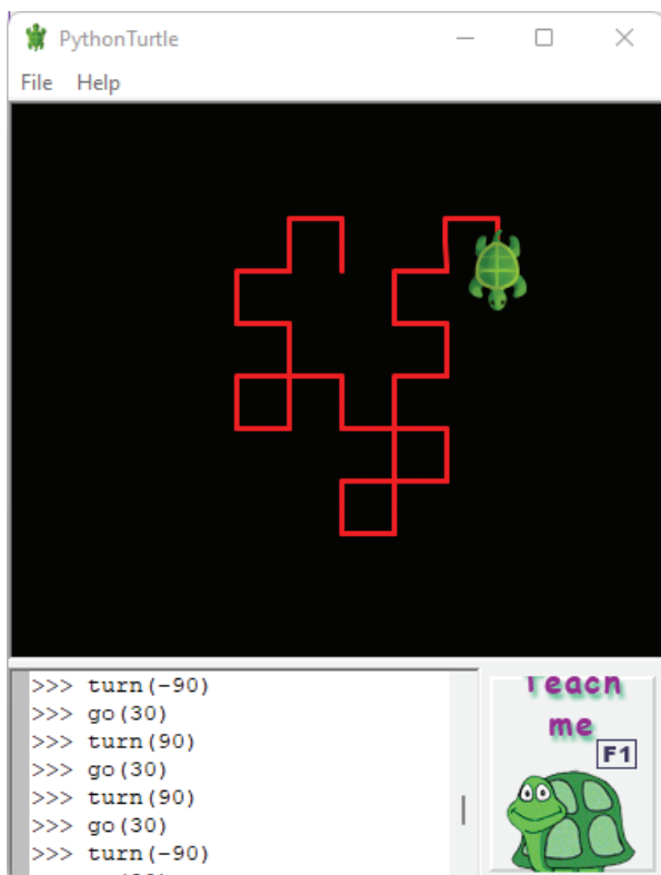
Jc'bx+#) I Početni segment zmajeve krivulje generirane L-sustavom
