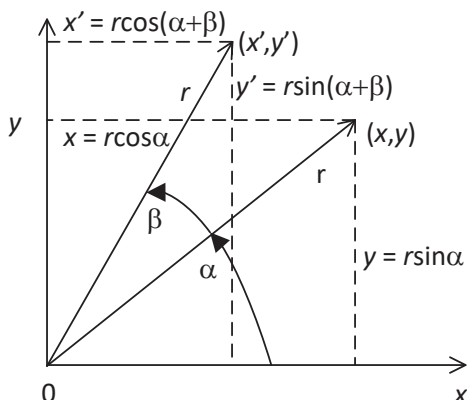
Jc`bX+{*I Vektor (x',y') u polarnom koordinatnom sustavu.
