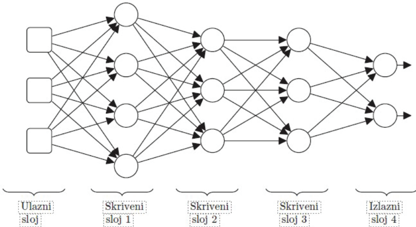
Jc`bX+#, IPrikaz višeslojnog perceptrona,preuzeto iz (Kelleher, 2021))
