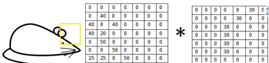
SLIKA 4-50: Konvolucija novog receptivnog polja sa starim filtrom.
