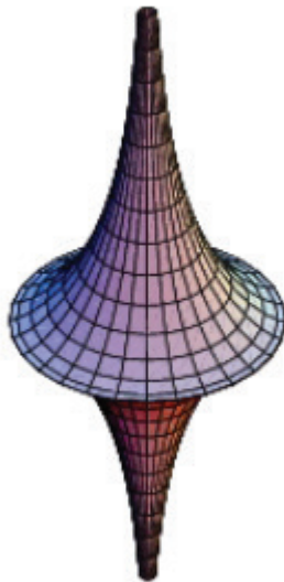
SLIKA 4-31: Pseudosfera-model hiperboličke geometrije.
